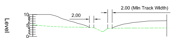
Combe Haven Cross Section 2 - 2 SCALE: H 1:500, V 1:500. DATUM: 0.000
