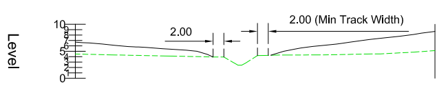
Combe Haven Cross Section 1 - 1 SCALE: H 1:500, V 1:500. DATUM: 0.000
