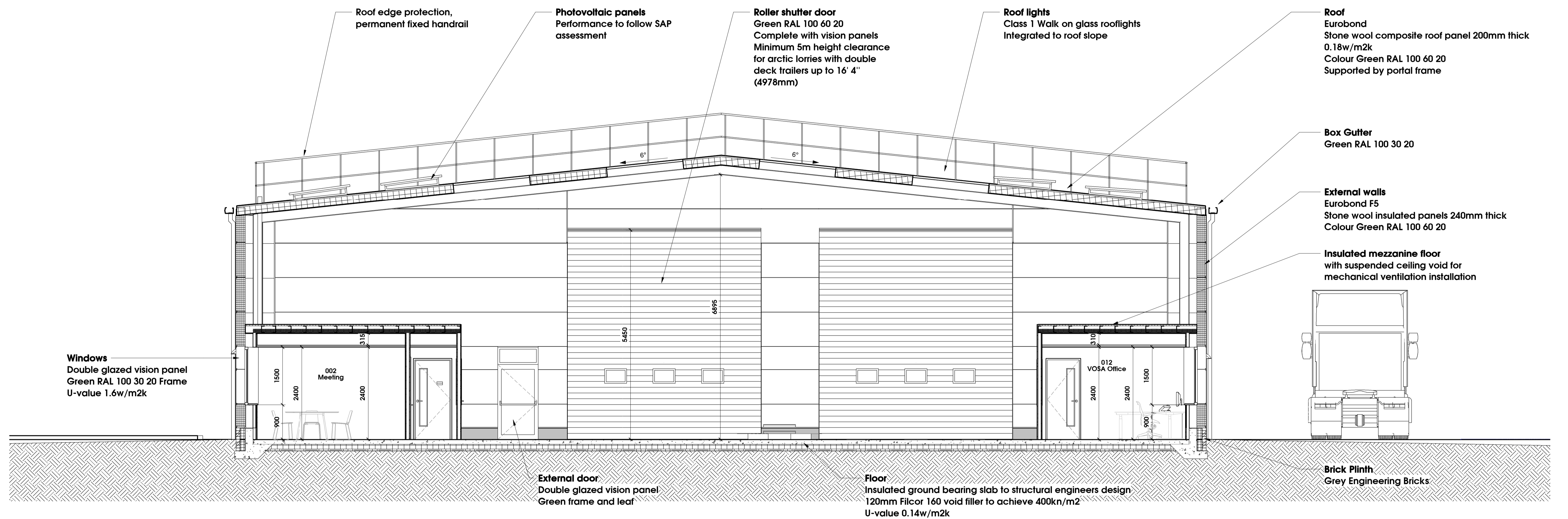
Section 1 1 : 50
